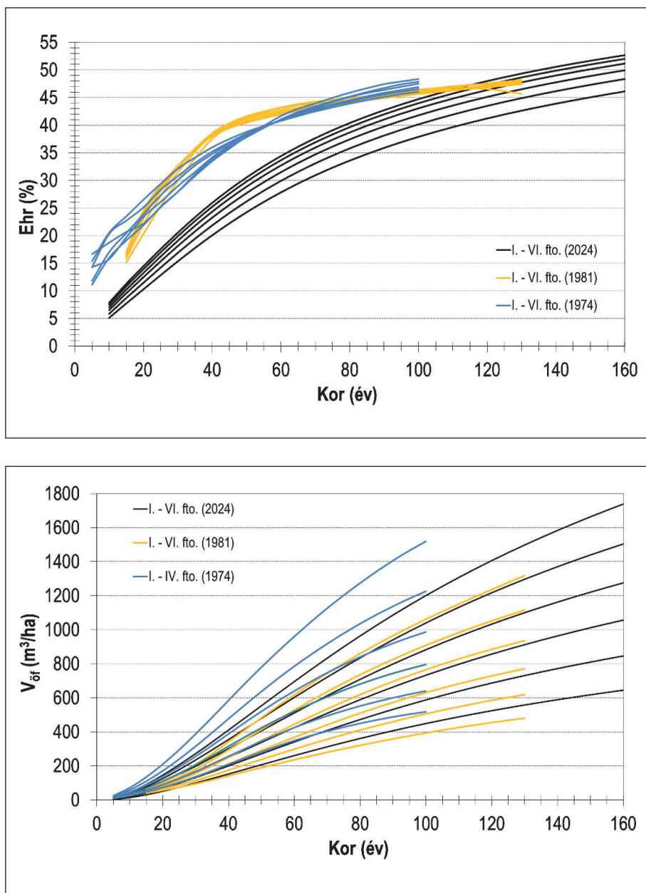
10. ábra: Az előhasználati részarány és az összes fatermés fatérfogata a kor függvényében ( E_{hr} , V_{\text{öf}} ), összehasonlítva az 1974-es (kék görbék) és 1981-es fatermési tábla adataival (sárga görbék) Figure 10: The intermediate cutting ratio and the total timber production depend on age ( E_{hr} , V_{\text{öf}} ), compare with the yield table data from 1974 (blue curves) and 1981 (yellow curves)
