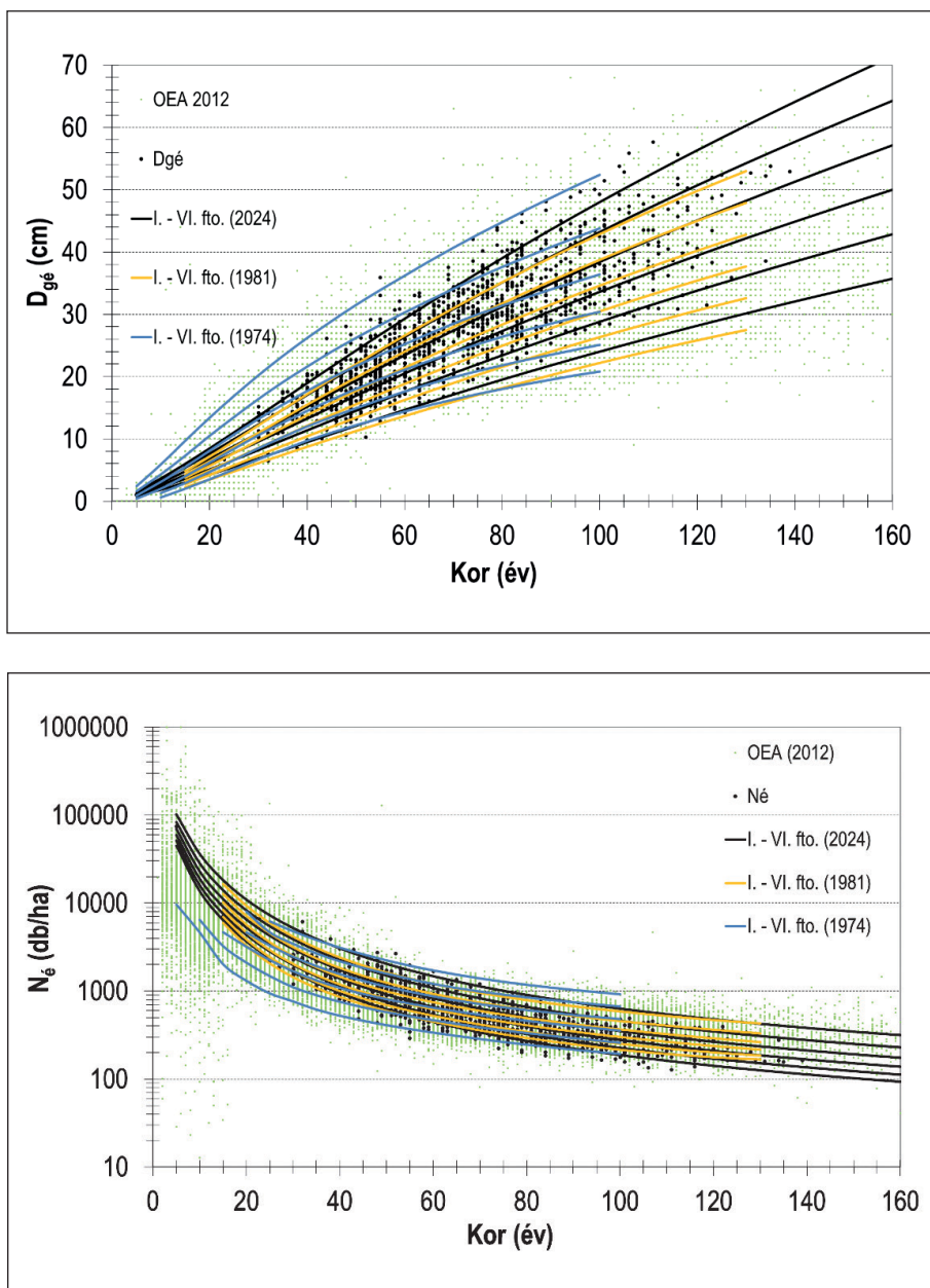
4. ábra: Az élőállomány átlagos átmérője és törzsszáma a kor függvényében ( D_{gé} , N_g ), összehasonlítva az 1974-es (kék görbék) és 1981-es fatermési tábla (sárga görbék) adataival. Az Országos Erdőállomány Adattár adatait (zöld pontok) is megjelenítettük
