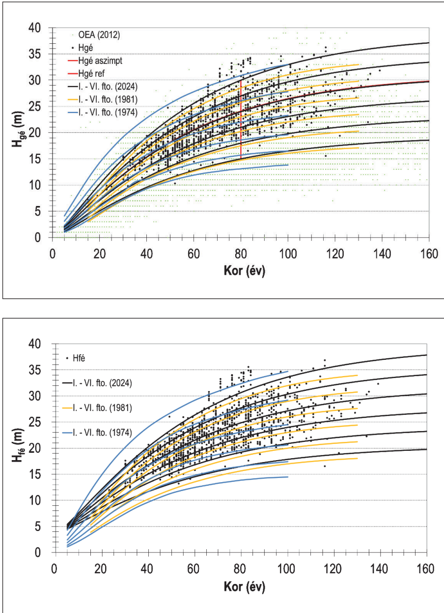
3. ábra: Az élőállomány átlagos és felső magassága a kor függvényében ( H_{gé} , H_{fé} ), összehasonlítva az 1974-es (kék görbék) és 1981-es fatermelési tábla adataival (sárga görbék). H_{gé} esetében az Országos Erdőállomány Adattár adatai (zöld pontok), az aszimptotikus vezérgörbe (piros görbe) és a 80 éves referenciakor magasság (piros függőleges vonal) is látható
