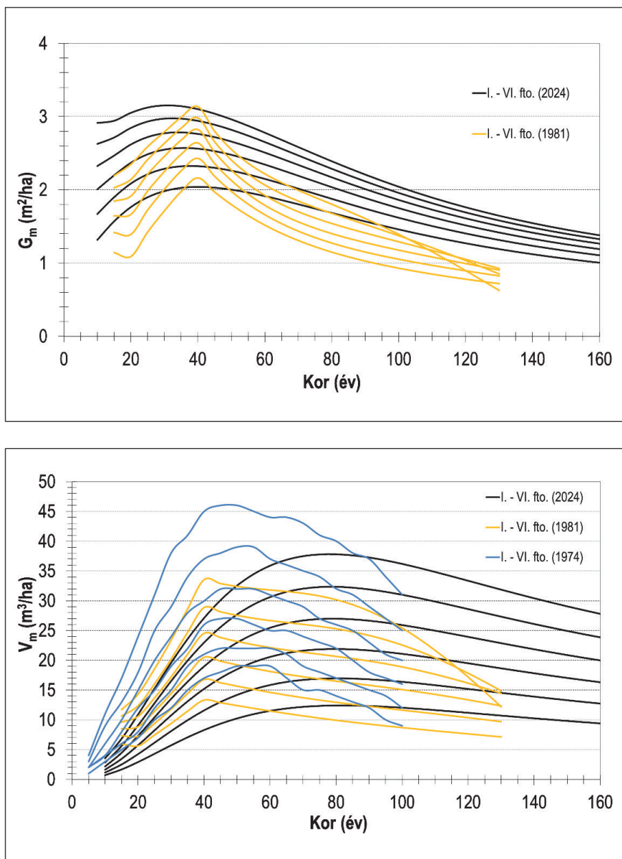
8. ábra: A mellékállomány körlapösszege és fatérfogata a kor függvényében ( G_m , V_m ), összehasonlítva az 1974-es (kék görbék, csak V_m ) és 1981-es fatermési tábla adataival (sárga görbék)
