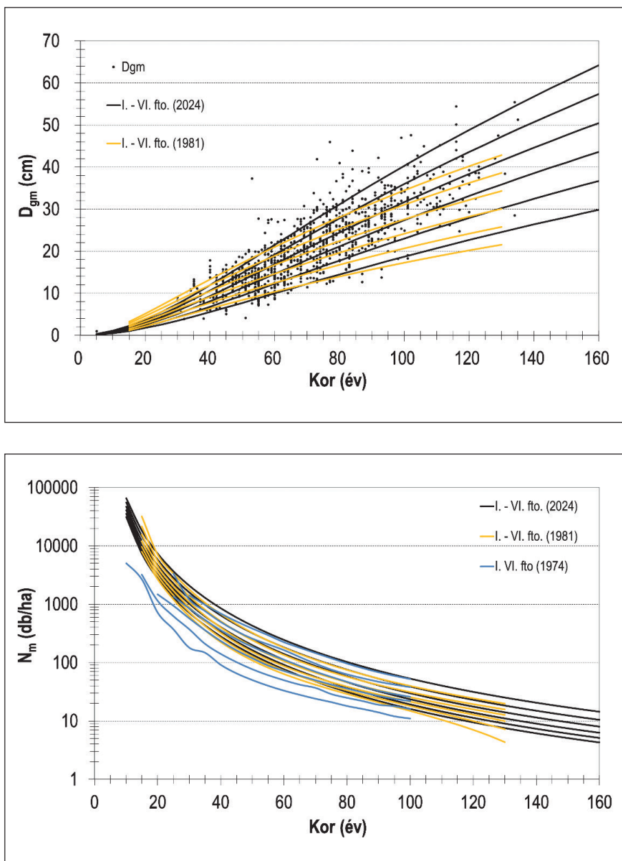
7. ábra: A mellékállomány átlagos átmérje és törzsszáma a kor függvényében ( D_{gm} , N_m ), összehasonlítva az 1974-es (kék görbék, csak N_m ) és 1981-es fatermési tábla adataival (sárga görbék) Figure 7: The average diameter and stem number for secondary stand depend on age ( D_{gm} , N_m ), compare with the yield table data from 1974 (blue curves, only N_m ) and 1981 (yellow curves)
