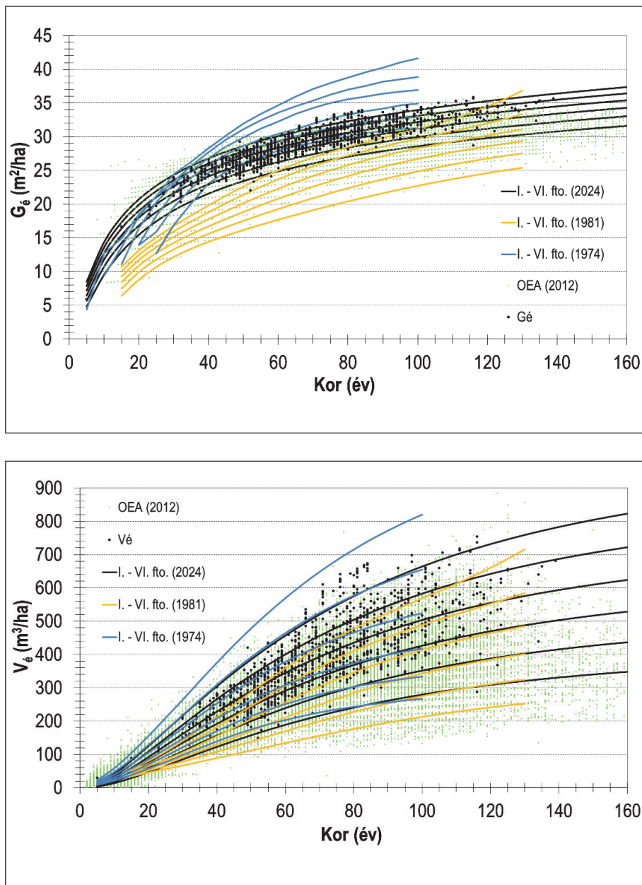
5. ábra: Az élőállomány körlapösszege és fatérfogata a kor függvényében ( G_e , V_e ), összehasonlítva az 1974-es (kék görbék) és 1981-es fatermési tábla (sárga görbék) adataival. Az Országos Erdőállomány Adattár adatait (zöld pontok) is megjelenítettük
