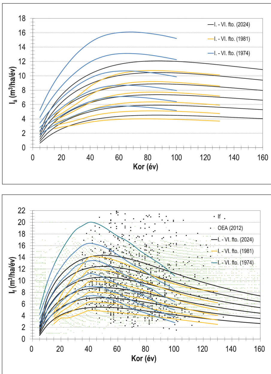
11. ábra: Az átlag- és folyónövedék a kor függvényében ( I_a , I_r ), összehasonlítva az 1974-es (kék görbék) és 1981-es fatermési tábla adataival (sárga görbék). I_r esetében az Országos Erdőállomány Adattár adatai (zöld pontok) is láthatóak
